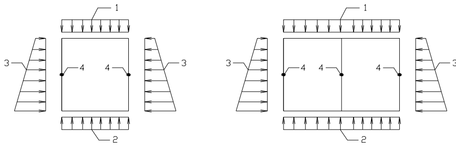
图 8.5.2-1 预制拼装综合管廊闭合框架计算模型
