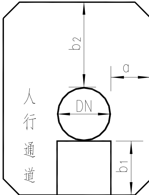
图 5.3.6 管道安装净距
