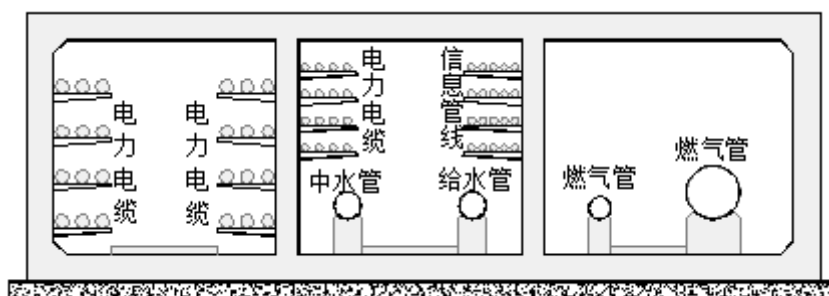
图 6 断面示意图 2
