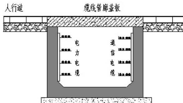
图 3 缆线综合管廊示意图
