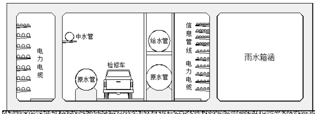
图 5 断面示意图 1
