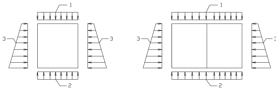
图 8.4.1-1 现浇综合管廊闭合框架计算模型
